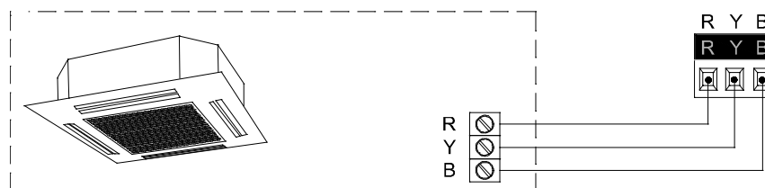
Figure 2. Câblage du KLIC-LG1 à l'appareil de climatisation
