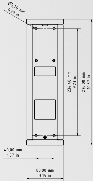
Boîtier de montage arrière (encastré)
