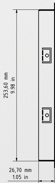
Boîtier de montage arrière (encastré)
