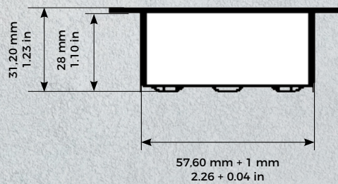
Boîtier de montage arrière (encastré)
