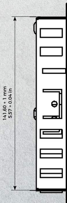
Boîtier de montage arrière (encastré)
