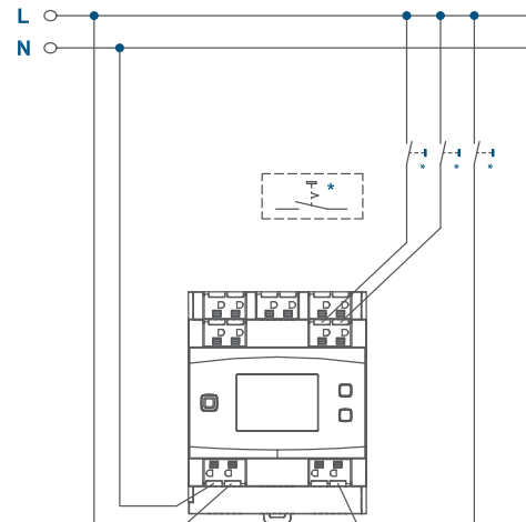
Raccordement de boutons-poussoirs/commutateurs (entrées) :
