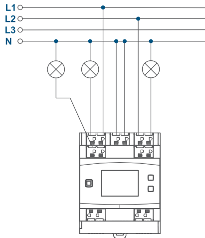
Raccordement de luminaires à intensité variable (sorties) :
