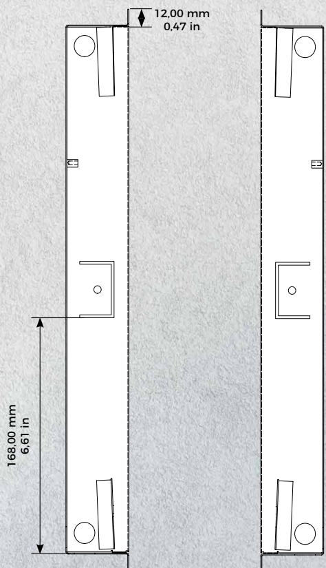
Unterputzgehäuse
