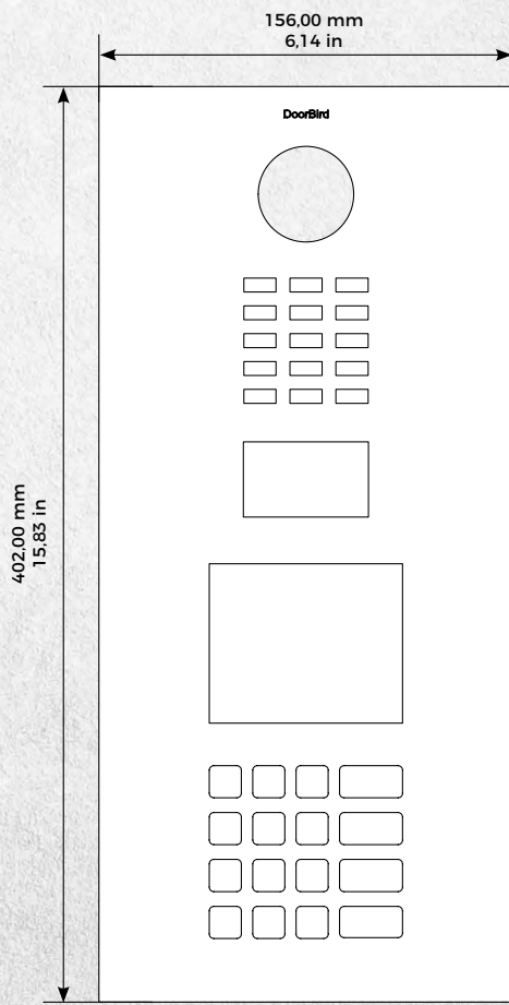
Frontblende
